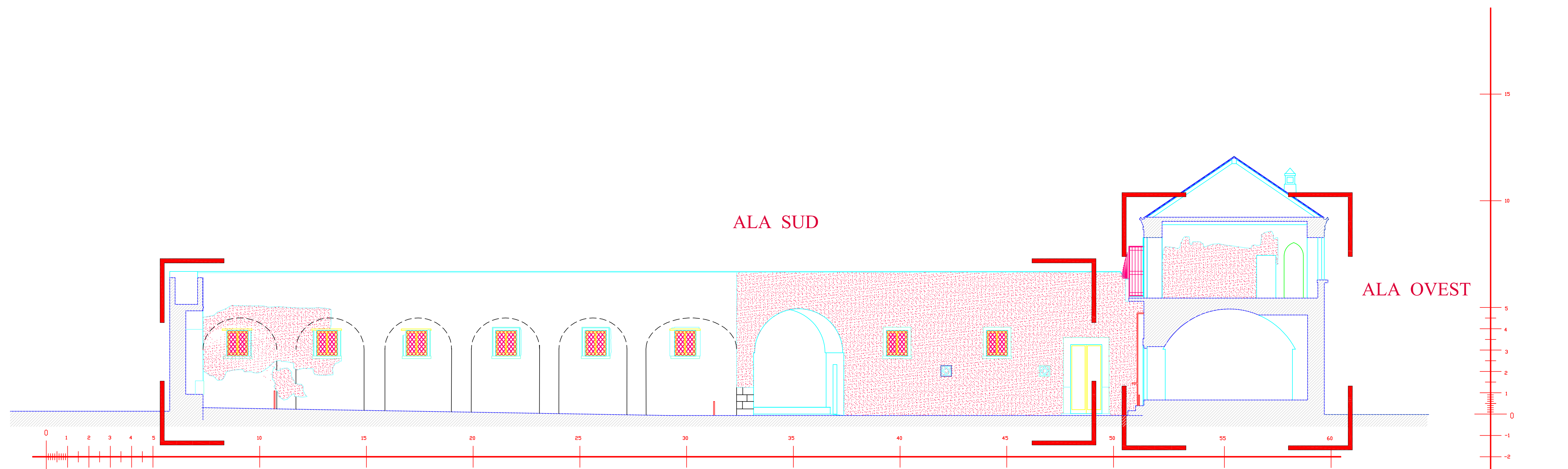
Prospetto Sud - Cortile Sez. E-E'
